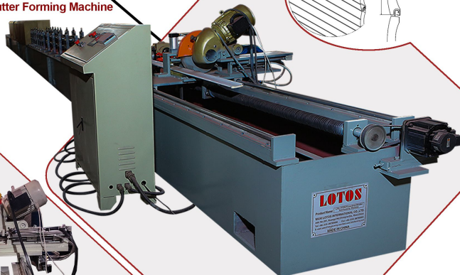
Pu Foam Door Shutter Forming Machine
